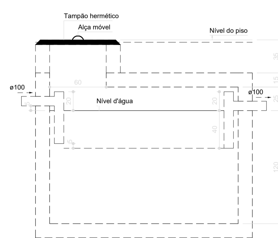
Tanque séptico Corte 1 - ESC. 1:25
